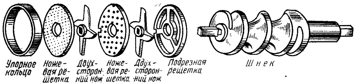
Мясорубка МИМ-500 (МИМ-105) (Основной набор ножей и решеток)
