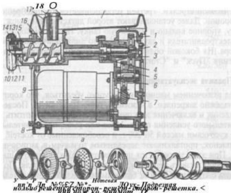
Рис. 4-1. Мясорубка МИМ-82.
