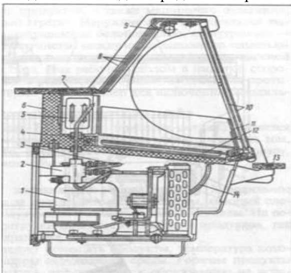
Рис. 15-5. Прилавок-витрина «Питтвин-В»:
