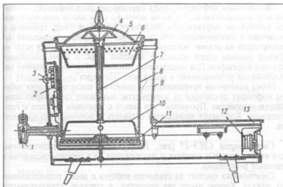
Рис. 10-3. Кофеварка КВЭ-7
